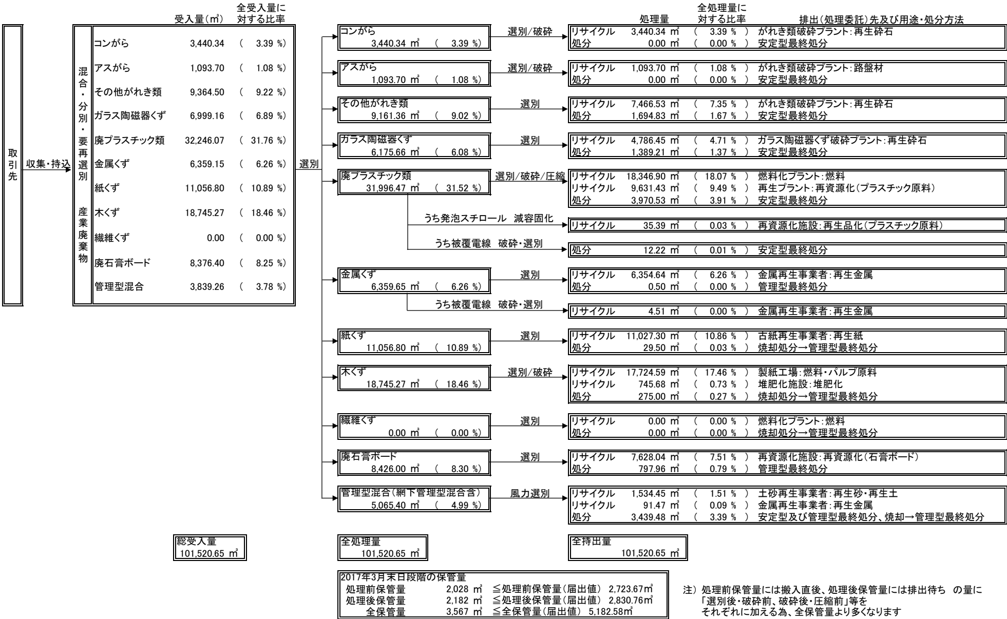
直前1年間(2017年4月～2018年3月)の産業廃棄物の一連の処理の行程
